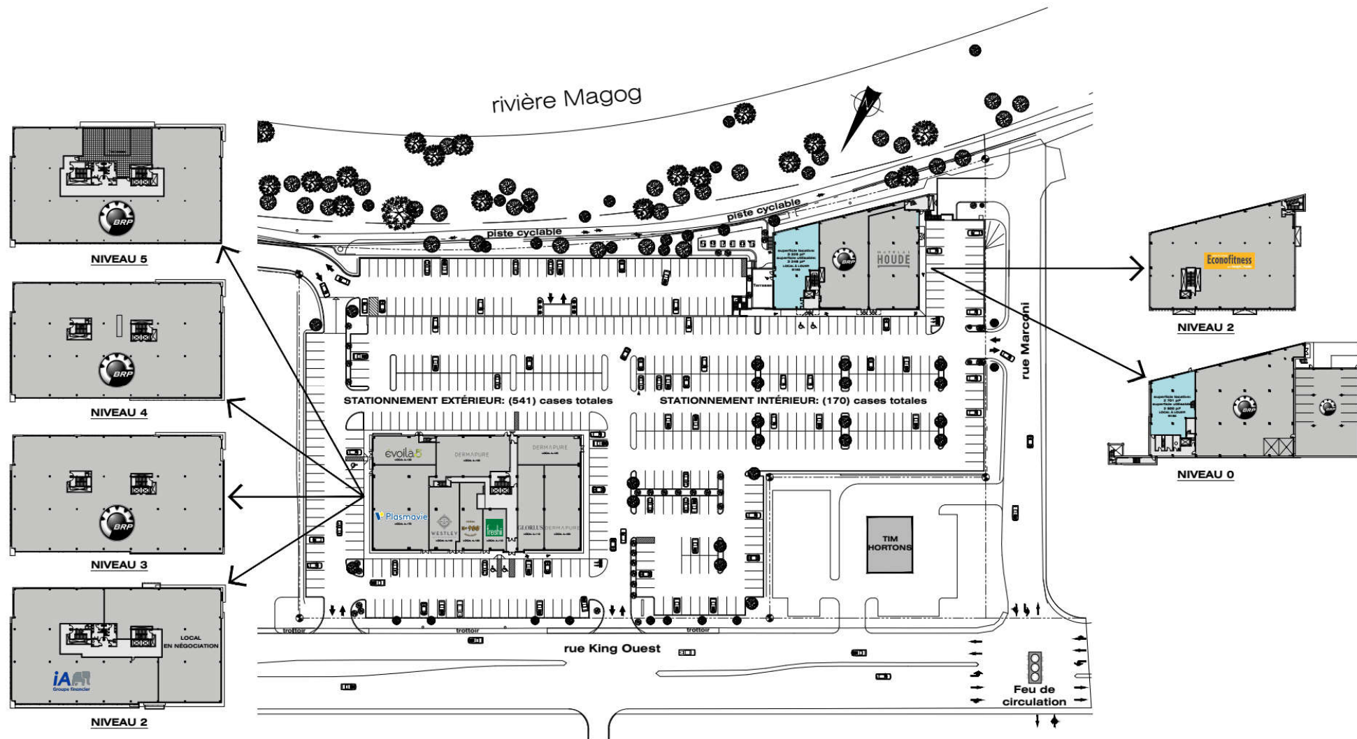
PLAN D'IMPLANTATION
