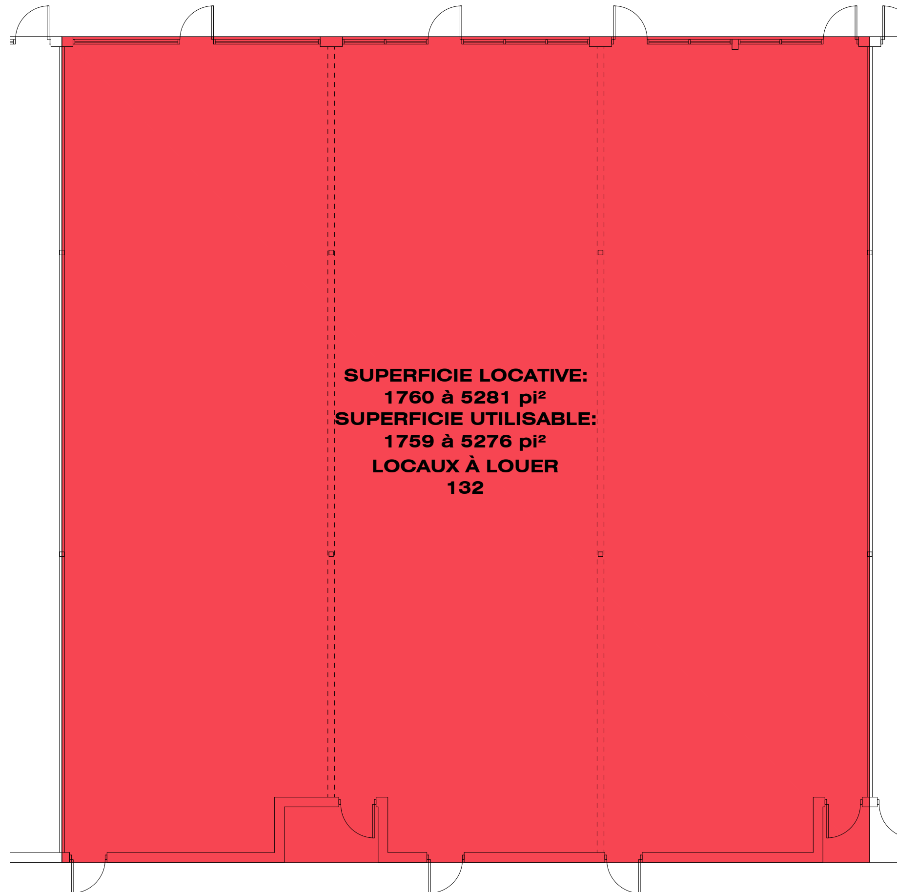
LOCAL 132 ÉCH: 1:100
